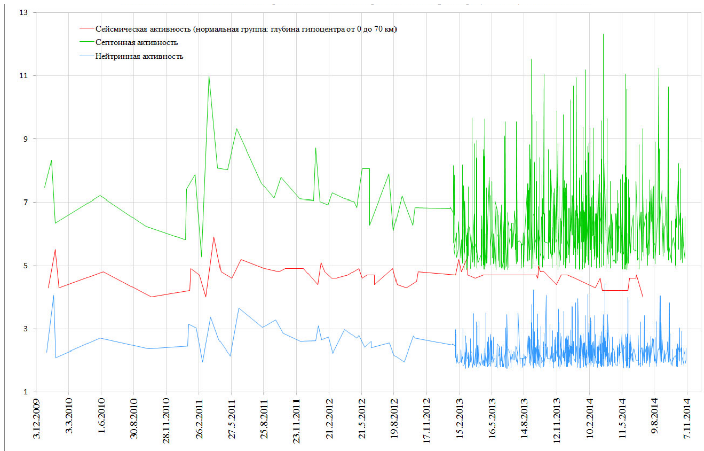
Сейсмическая, септонная и нейтринная активность в районе кальдеры Айра (Япония) с 2010-2014 гг.
