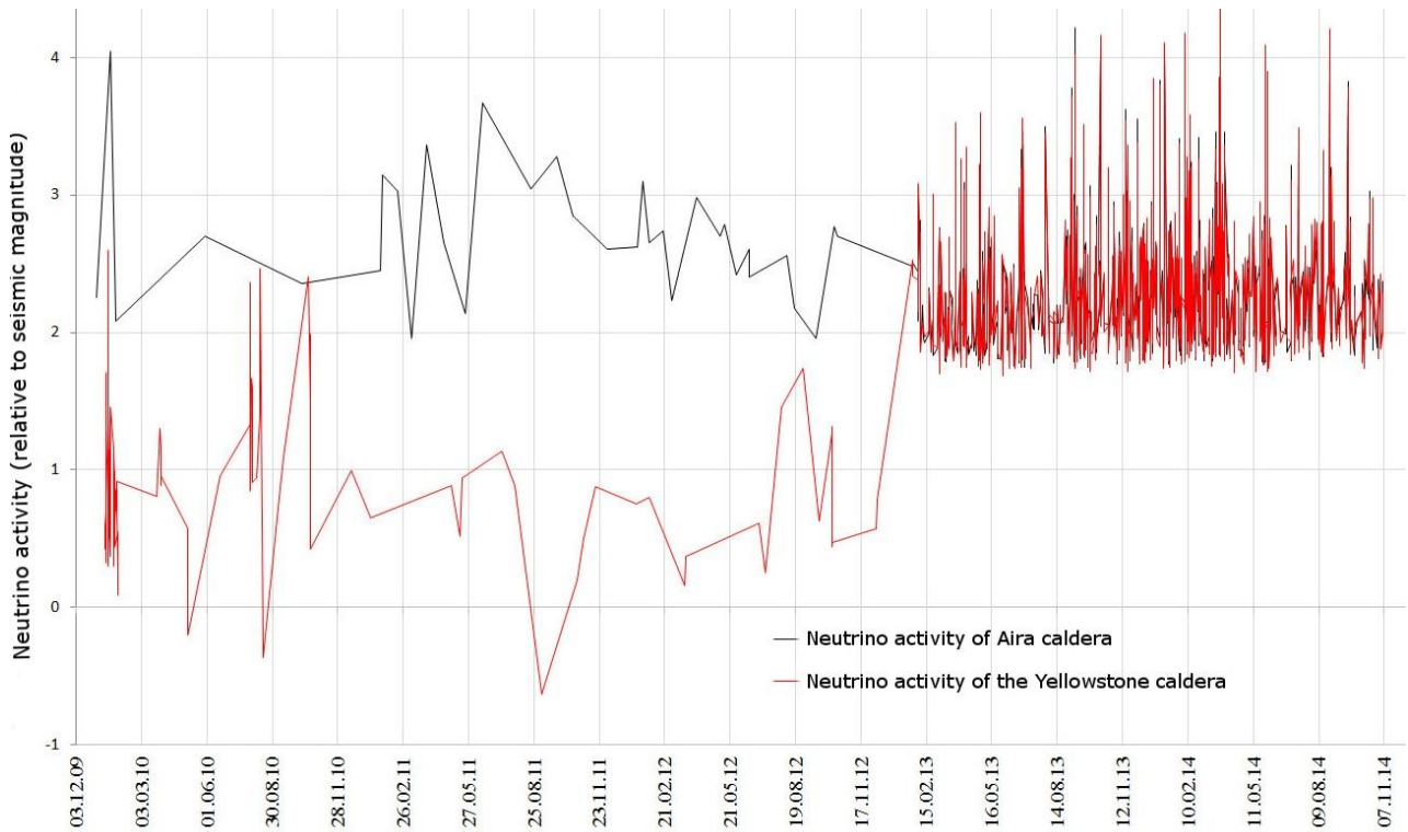
2010~2014 년 칼데라 옐로우 스톤 (미국) 뉴트리노 활동
