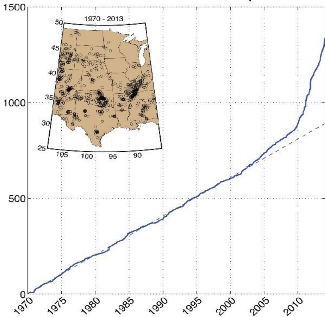
1970~2013년 간 북미 지역에 발생 지진 수 (>3도 강도)
