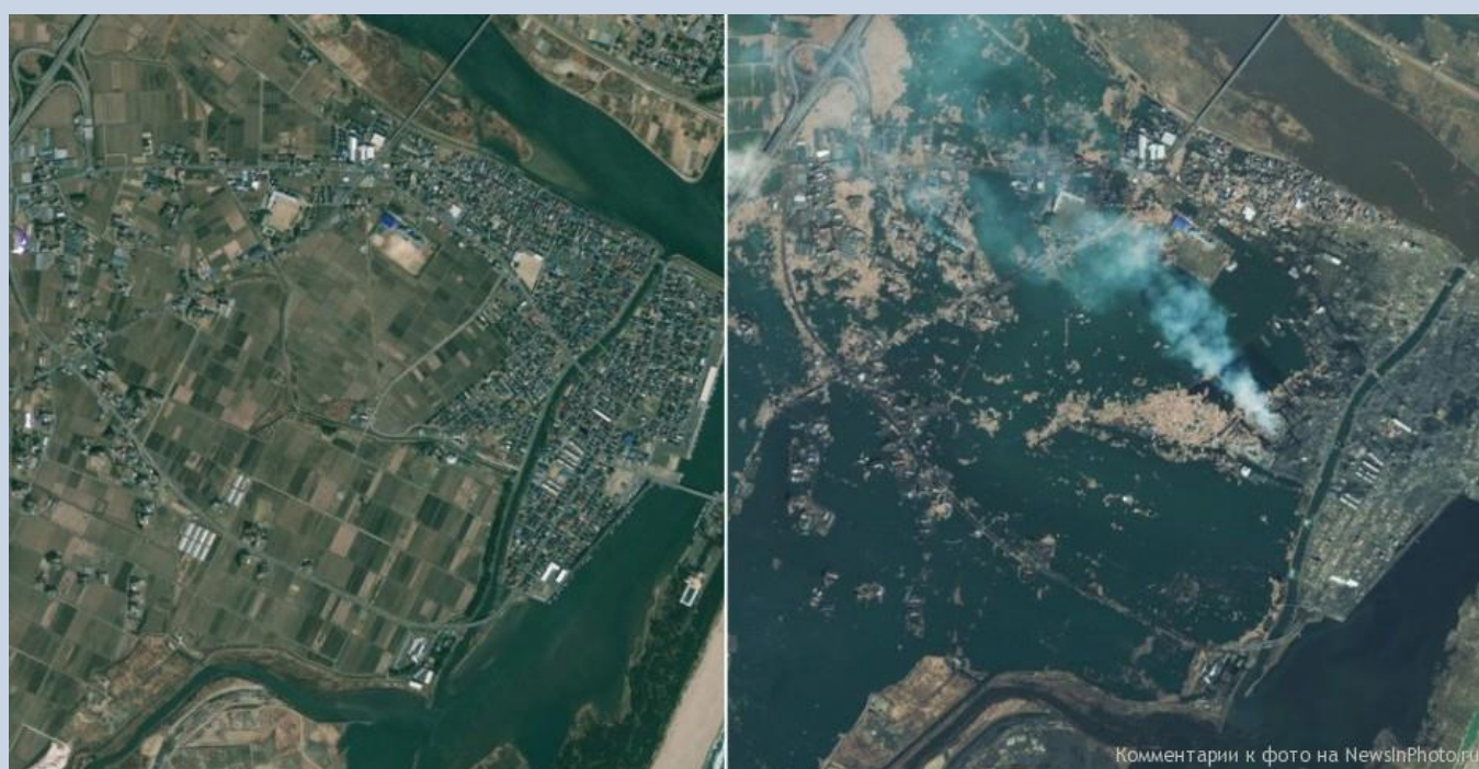
나토리 일본 도시 사진: 8.9도 강도의 지진 발생 이전 (좌) 및 발생 이후 (우). 본 지진은 2011년 3월 11일 오시카 반도에서 발생. 출처: Geo Eye Corporation
