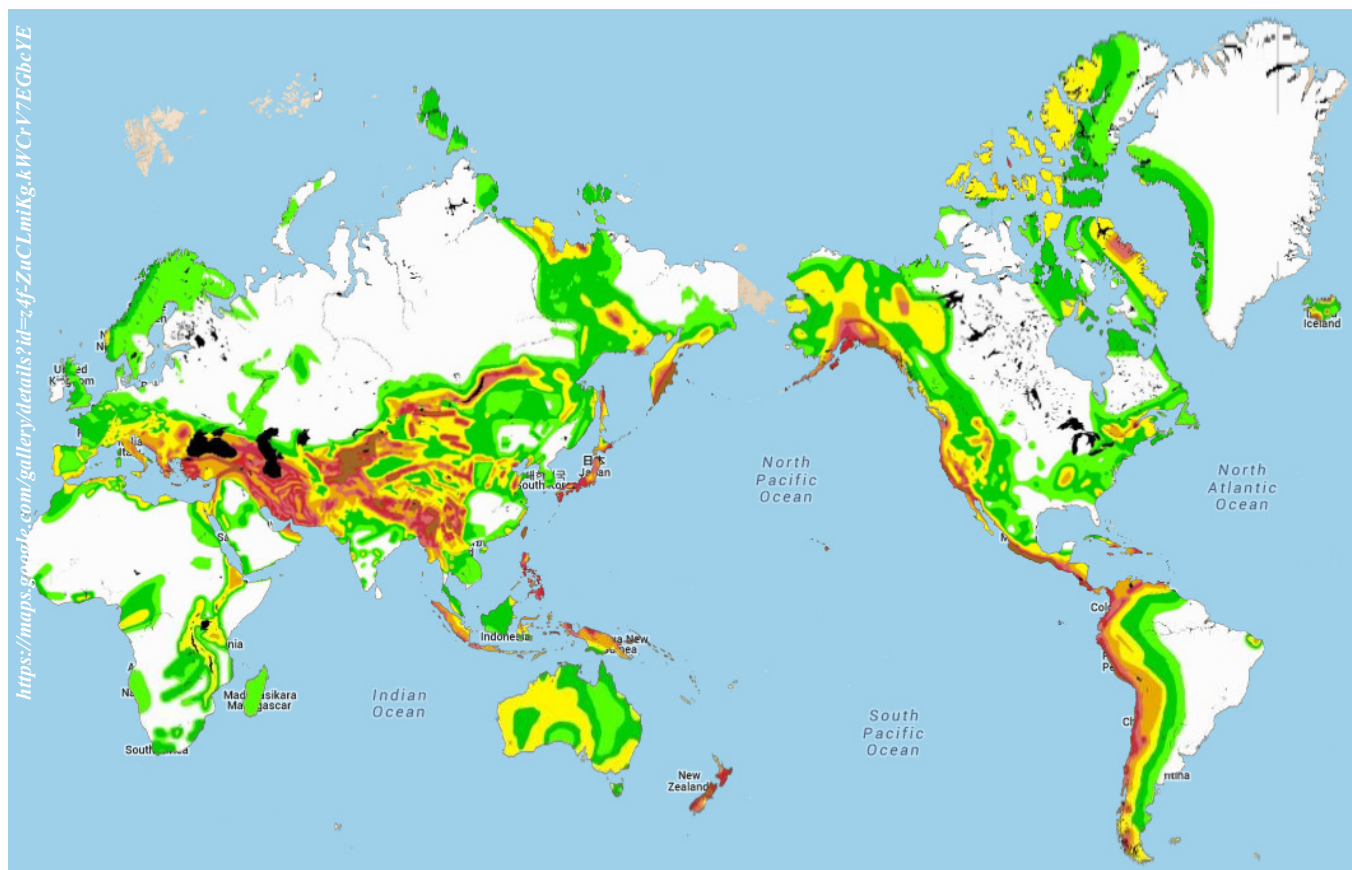
Mapa globálního seismického ohrožení pro rok 2014
