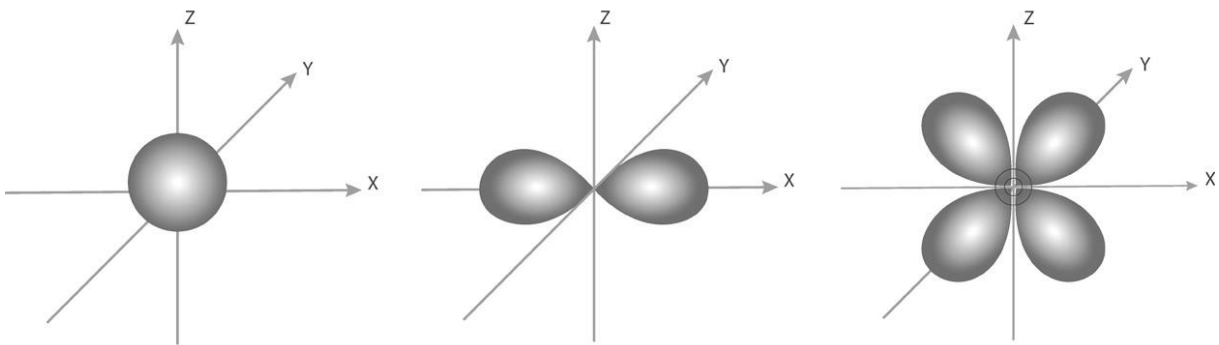
Şekil 3. Atomik yörüngelerin çeşitli şekilleri (kuantum kimyanın "geometrisi").
