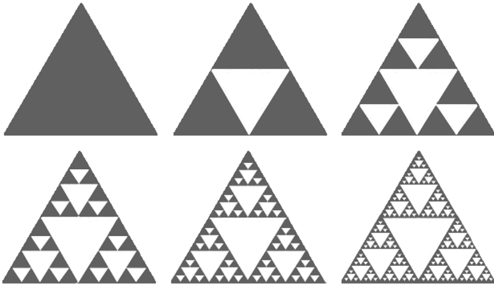
Şekil 65. Sierpinski Fraktal üçgeni. Dört eşit eşkenarlı üçgen tarafından bölünmenin sürekli tekrarlanması ile üçgenin içinde bir fraktal inşa etme işlemi.
