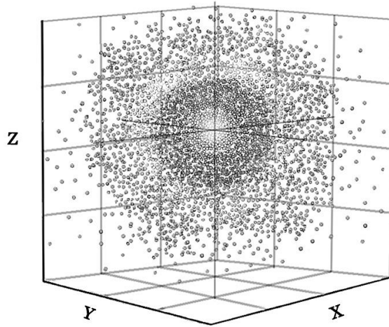
Şekil 2. Hidrojen atomunun elektron bulutu: elektronun en muhtemel yerini koruyan atom çekirdeği etrafındaki üç boyutlu uzay bölgesi.
