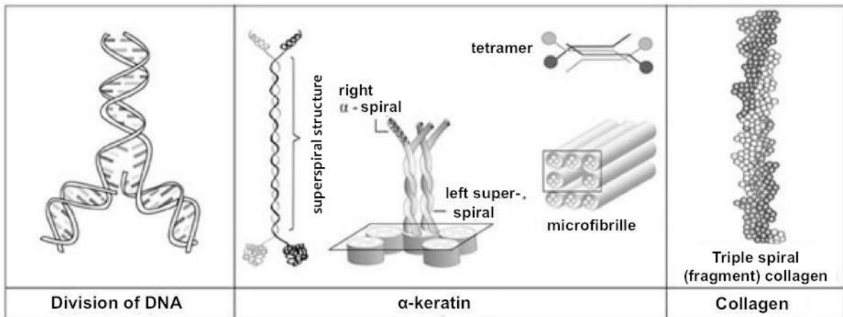
Şekil 1. Sarmal yapılar:
