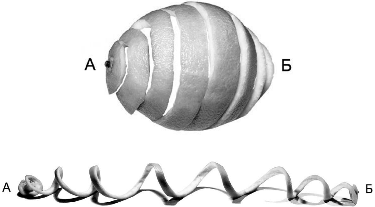
Şekil 4. Elektronun parçacıktan dalgaya dönüşümünün temsili örneği: 1) parçacık hali; 2) dalga hali.
