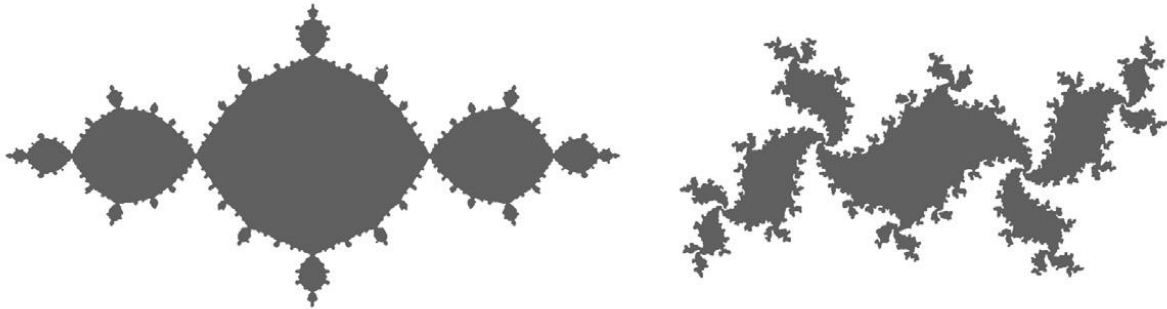
Şekil 64. Julia Seti
