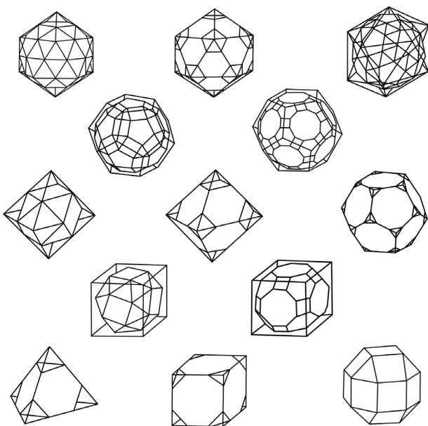
Slika 60. Izvorna postavitev 13 polpravilnih poliedrov.
