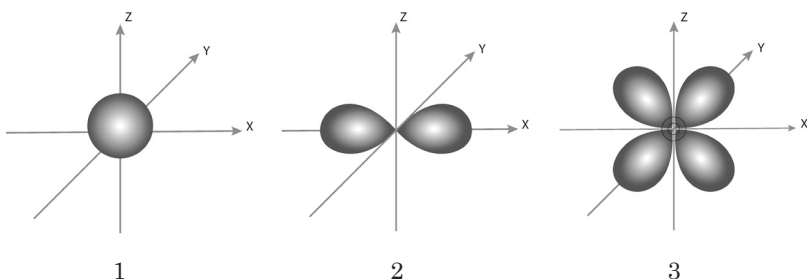
Slika 3. Različne oblike atomskih orbital
