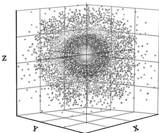
Slika 2. Elektronski oblak vodikovega atoma: področje tridimenzionalnega prostora okrog atomskega jedra, ki prikazuje najverjetnejše lokacije elektrona.
