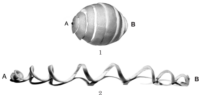
Slika 4. Metaforičen primer preobrazbe elektrona iz delca v val:
