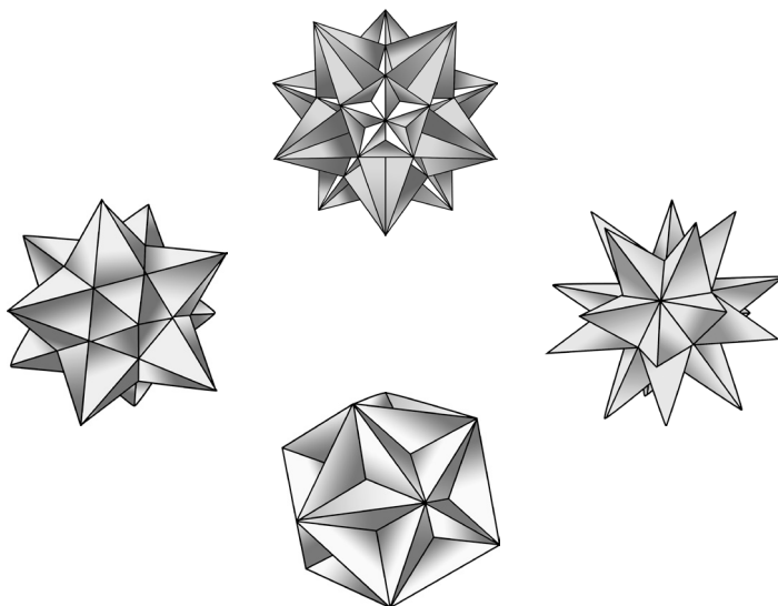
Slika 62. Zvezdni poliedri: Kepler-Poinsotova telesa.
