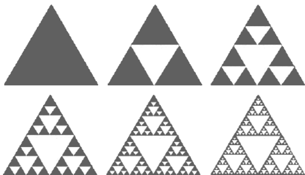
Obrázok 65. Fraktál „Sierpiňského trojuholník“
