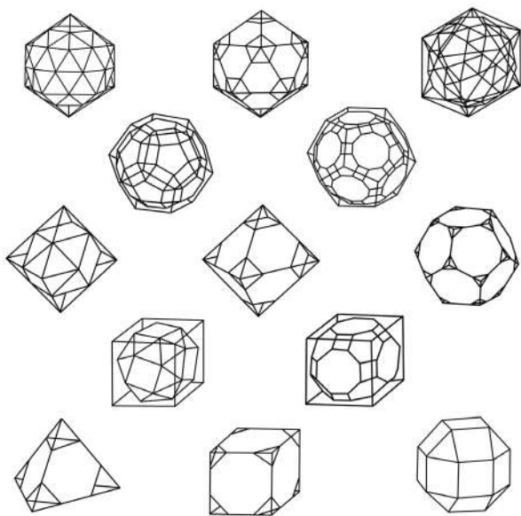
Obrázok 60. Prapôvodná schéma rozmiestnenia 13-tich poloprávdelných mnohostenov
