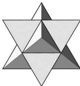
Obrázok 61. Hviezdicový osemsten (oktaeder) Leonardo da Vinci
