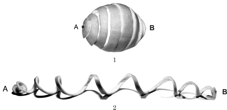
Figura 4. Exemplu figurativ de transformare a electronului dintr-o particulă într-o undă:
