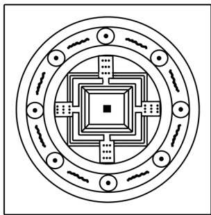
Figura 71. Mandala și yantra.
