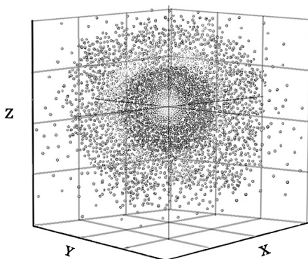
Figura. 2. Norul de electroni al atomului de hidrogen:
