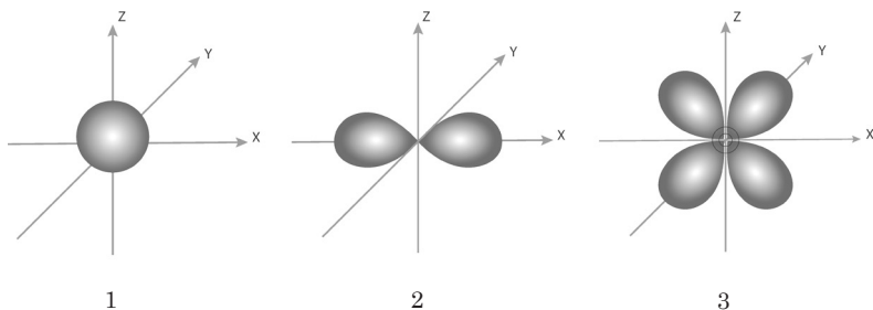
Figura 3. Forme variate ale norului de electroni („geometria” chimiei cuantice)
