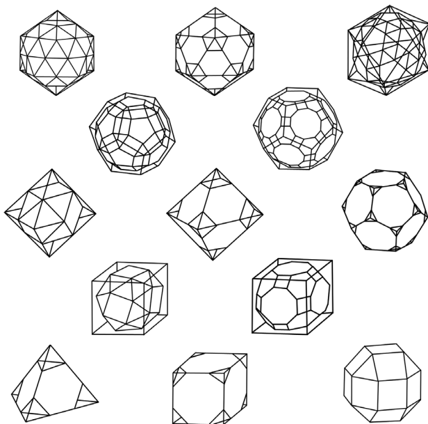
Figura 60. Aranjamentul primordial al celor 13 poliedre semiregulate.
