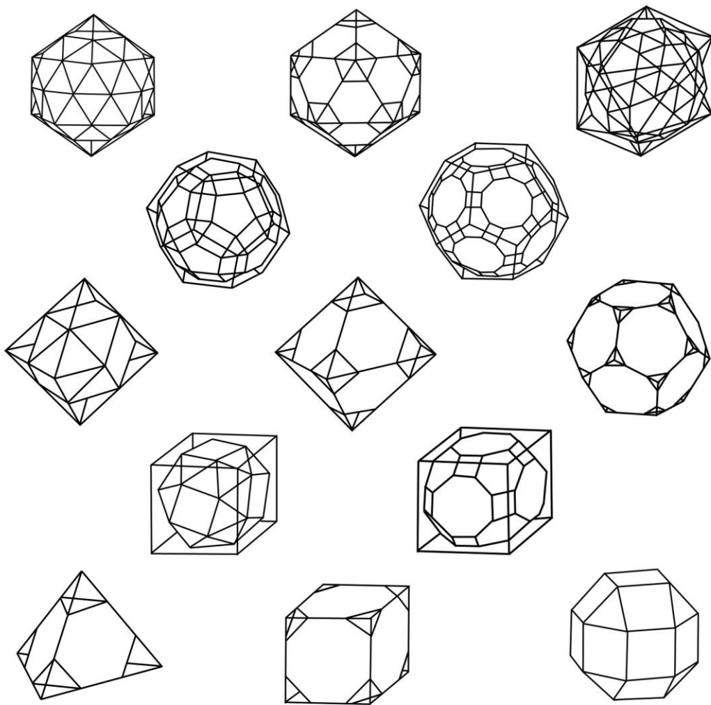
Figuur 60. De oorspronkelijke rangschikking van 13 halfregelmatige veelvlakken.
