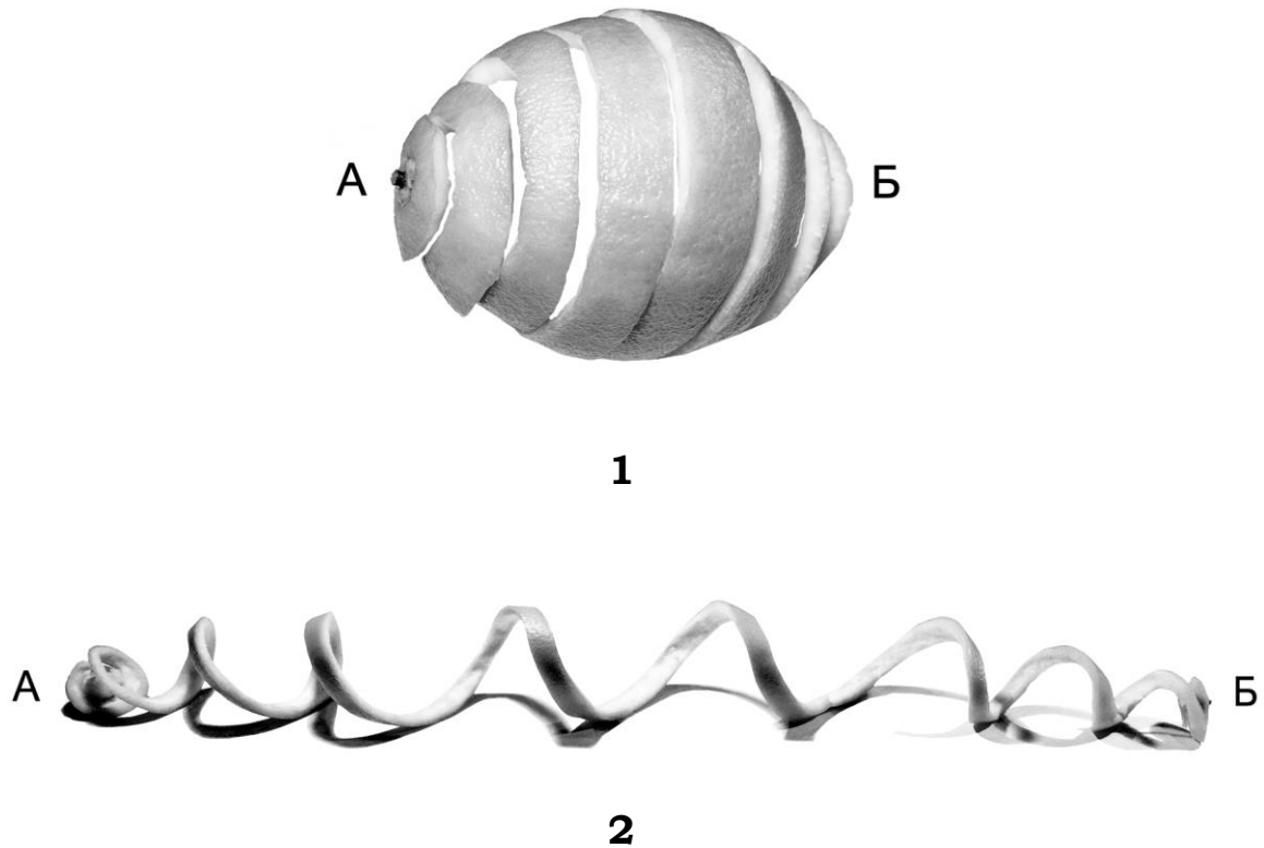
Figuur 4. Een figuratief voorbeeld van de elektronentransformatie van een deeltje in een golf:
