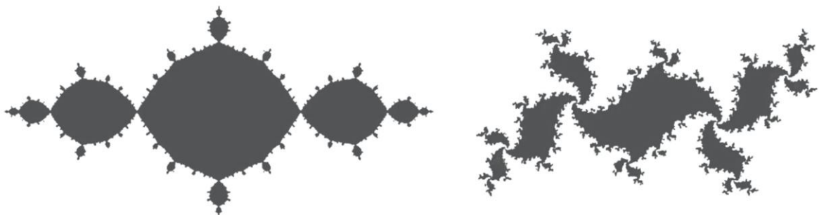
Figuur 64. Juliaverzameling.
