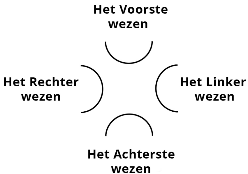
Figuur 33. Schematische aanduiding van de Wezens van de mens als bogen.
