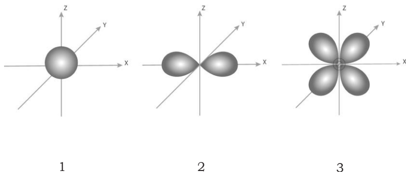
Slika 3. Različiti oblici atomskih orbitala („geometrija“ kvantne kemije)
