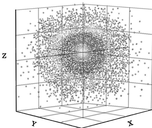
Slika 2. Elektronski oblak atoma vodika: područje trodimenzionalnog prostora oko jezgre atoma koje zauzima najvjerojatniju lokaciju elektrona
