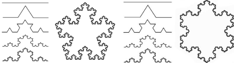
Slika 66. Kochov fraktal snopa snježne pahulje.
