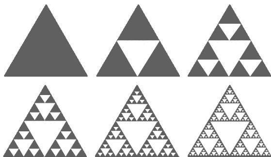
Рисуника 65. Фракталът "Триъгълник на Серпински".
