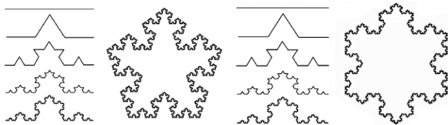
Рисуника 66. Фрактал "Снежинката на Кох". Два примера за процеса на превръщане на линия в снежинка по пътя на многократно разделяне на сегмент на линия на три равни части и замяна на средната част с два нови сегмента с аналогична дължина.
