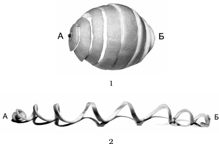
Рисуника 4. Образен пример за преобразуване на електрона от частица във вълна: 1) състояние на частица; 2) състояние на вълна
