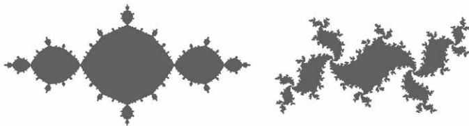
Рисунка 64. Множеството на Жюлиа.
