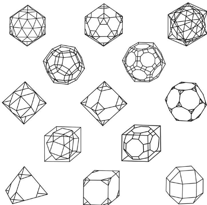
Рисуника 60. Изконна схема на разположение на 13-те полуправилни многостенници.
