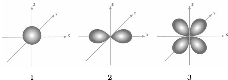
Рисуника 3. Различни форми на електронния облак ("геометрия" на квантовата химия):
